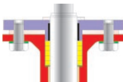
Bild 1 - Edelstahl-Stellklappe BR 14 mit nachstellbarer Stopfbuchse
