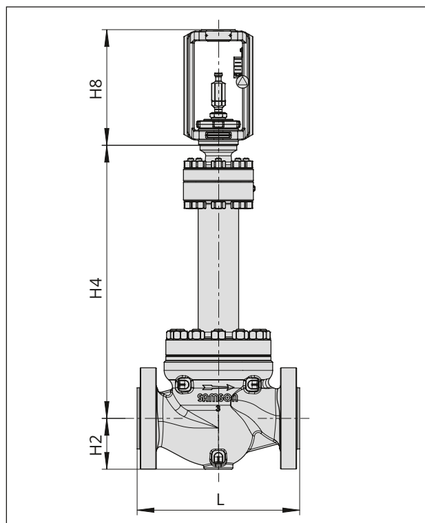
Bild 8: Ventil Typ 251GR in Ausführung mit Balgteildichtung
