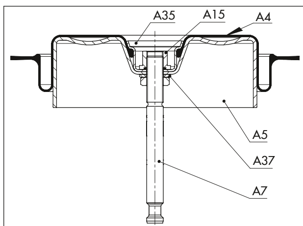
图 16: 针对“推杆缩回”动作方向的部件排列
