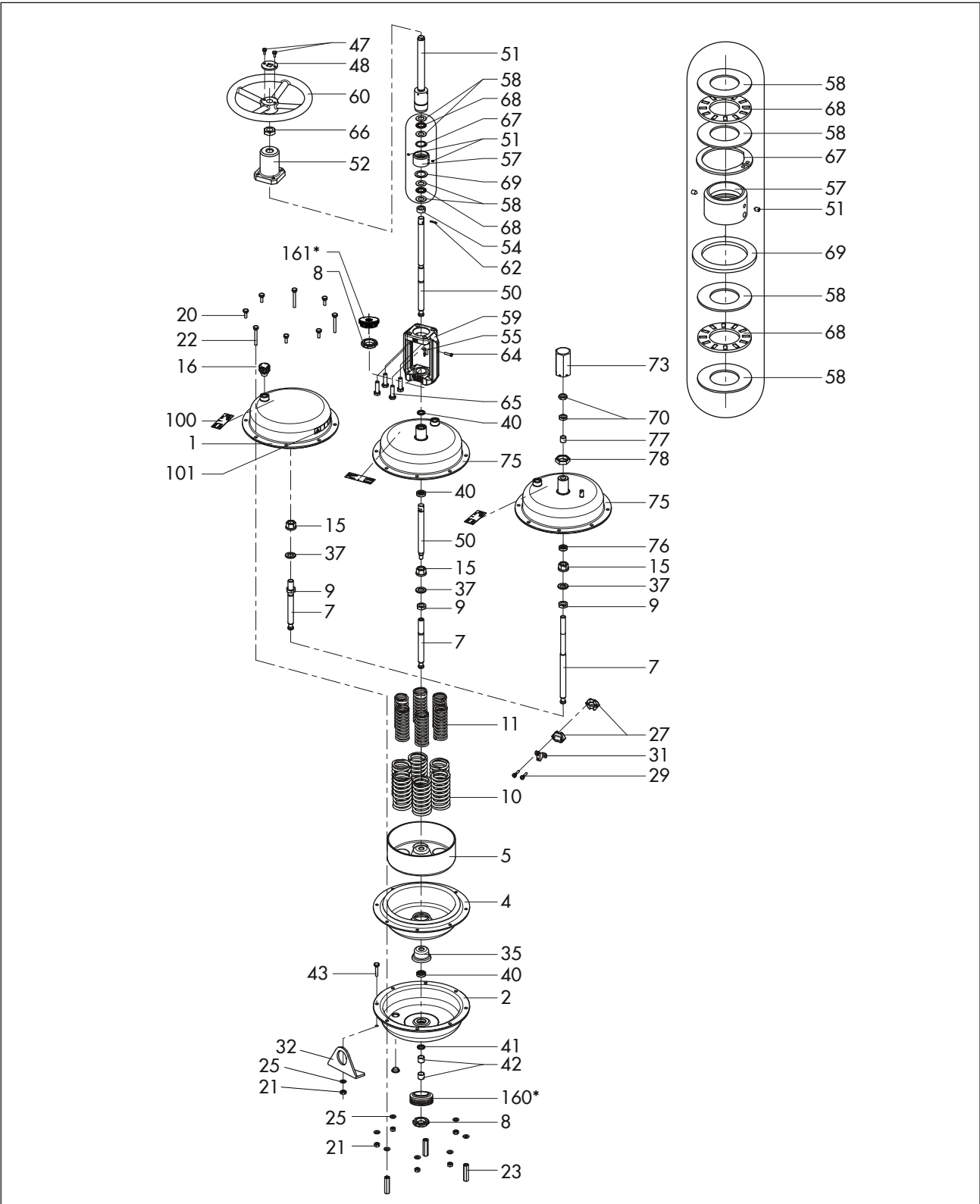
图 21: 3271 型执行机构 (355v2 cm²)
