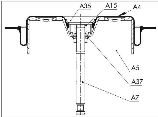
图 18: 针对“推杆缩回”动作方向的部件排列
