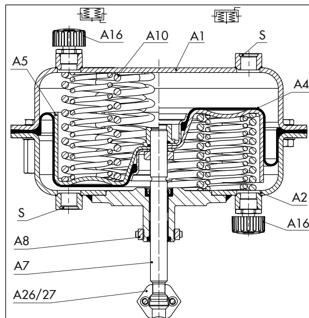
图 2: 3271 型执行机构，显示了 355v2 cm 2 执行机构面积示例的绘图
