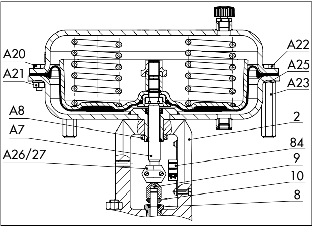
图 12: 单座直通阀上安装的 3271 型气动执行机构
