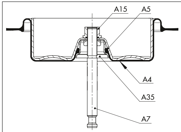
图 19: 针对“推杆伸出”动作方向的部件排列
