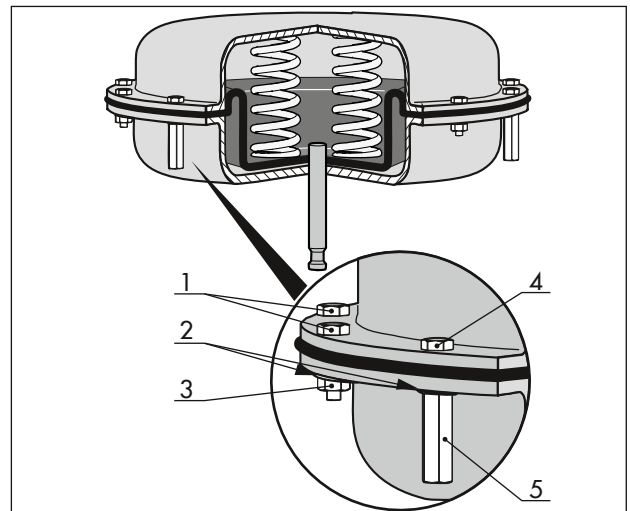
图 20: 预加载弹簧（功能图）
