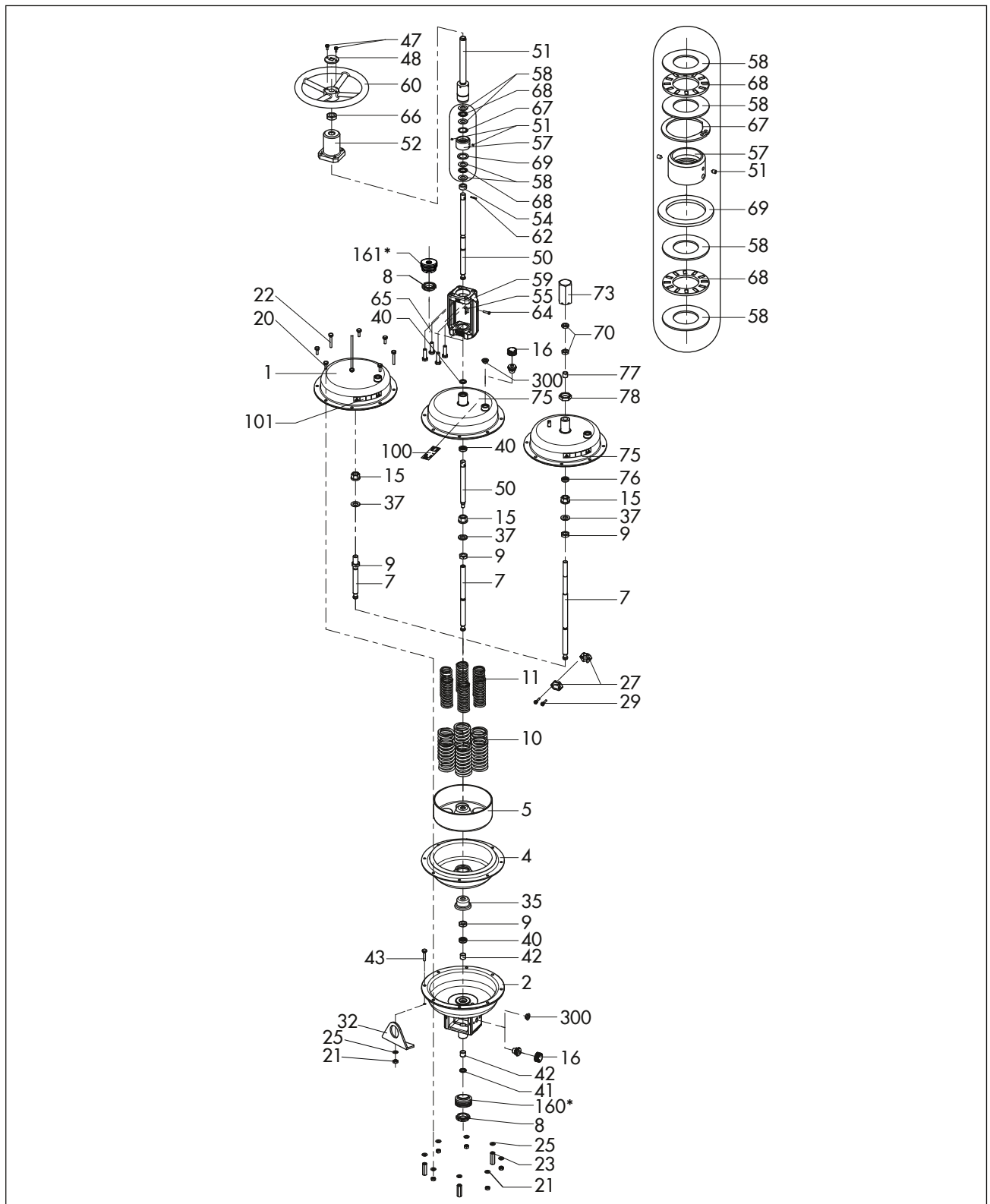
图 22: 3277 型执行机构 (355v2 cm 2 )
