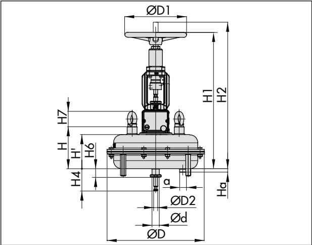
图 5: 两侧带手轮和行程限位的 3271 型气动执行机构
