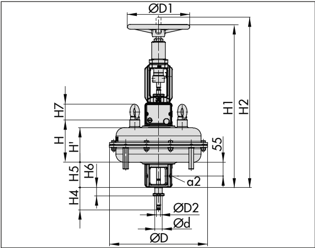
图 8: 两侧带手轮和行程限位的 3277 型气动执行机构
