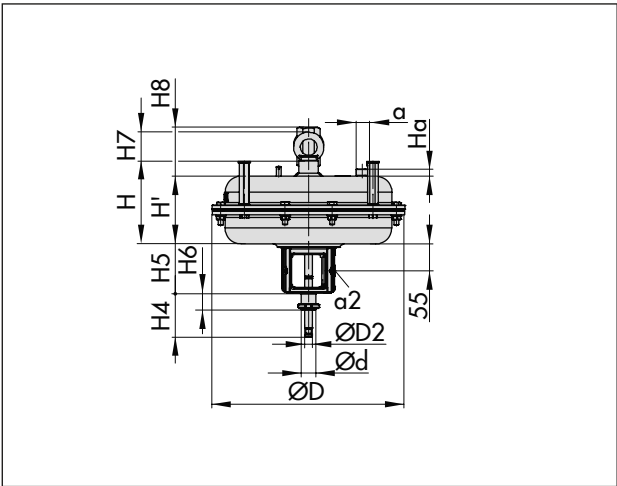
图 9: 3277 型, 带行程限位
