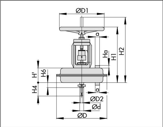
图 4: 3271 型，带额外手轮
