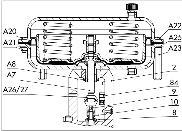
图 10: 单座直通阀上安装的 3271 型气动执行机构
