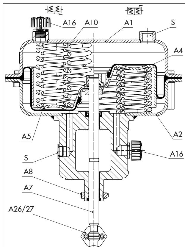
图 3: 3277 型执行机构，显示了 355v2 cm 2 执行机构面积示例的绘图
