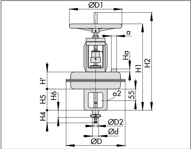
图 7: 3277 型，带额外手轮
