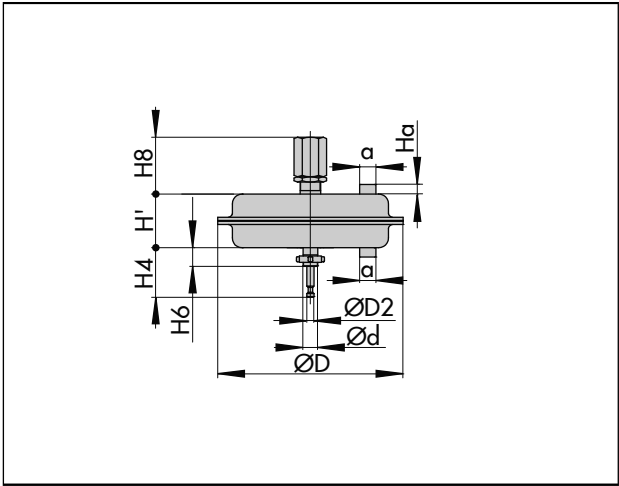
图 6: 3271 型，带行程限位
