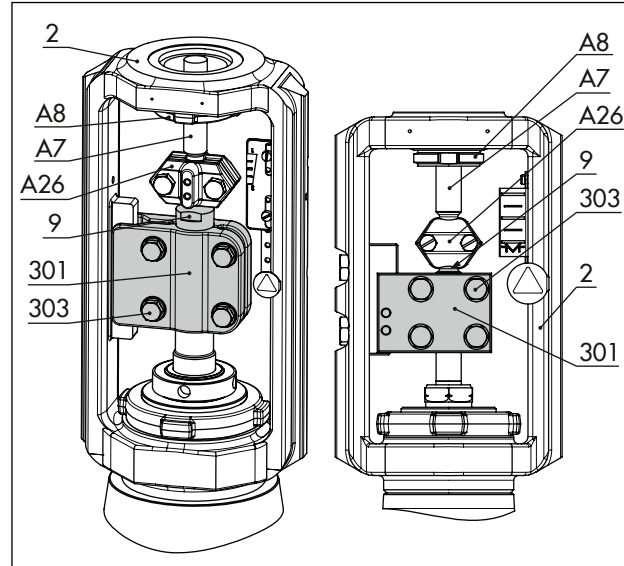
图 11: 防旋转夹具：标准类型（左侧）和特殊类型（右侧）
