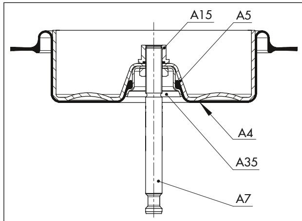
图 15: 针对“推杆伸出”动作方向的部件排列
