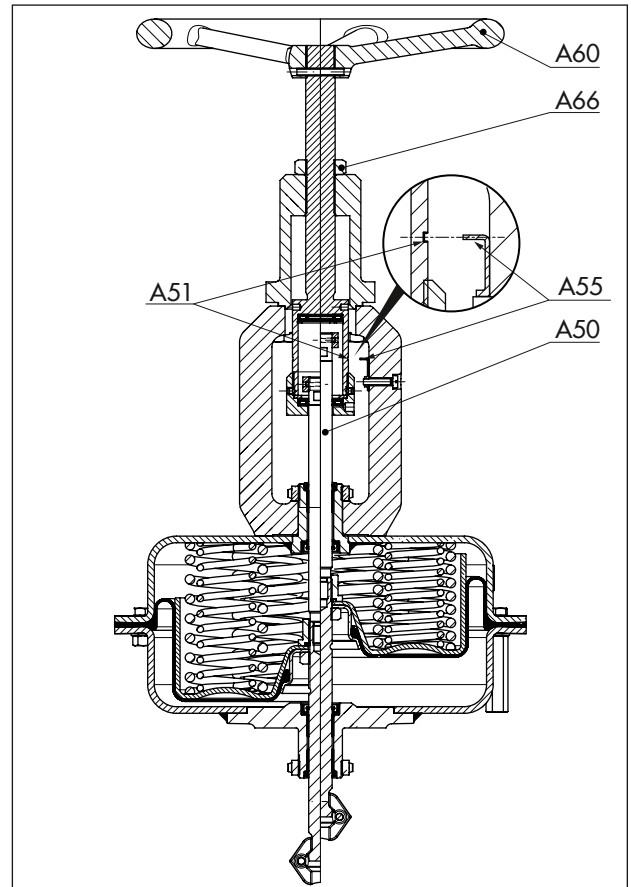
图 14: 带手轮的 3271 型执行机构 (355v2 cm 2 )
