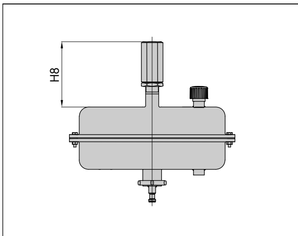
Fig. 4: Superficie de accionamiento 1400-60 cm 2 , con limitación de carrera ajustable
