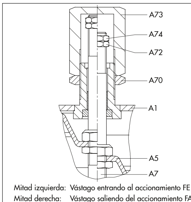
Fig. 11: Limitación de carrera
