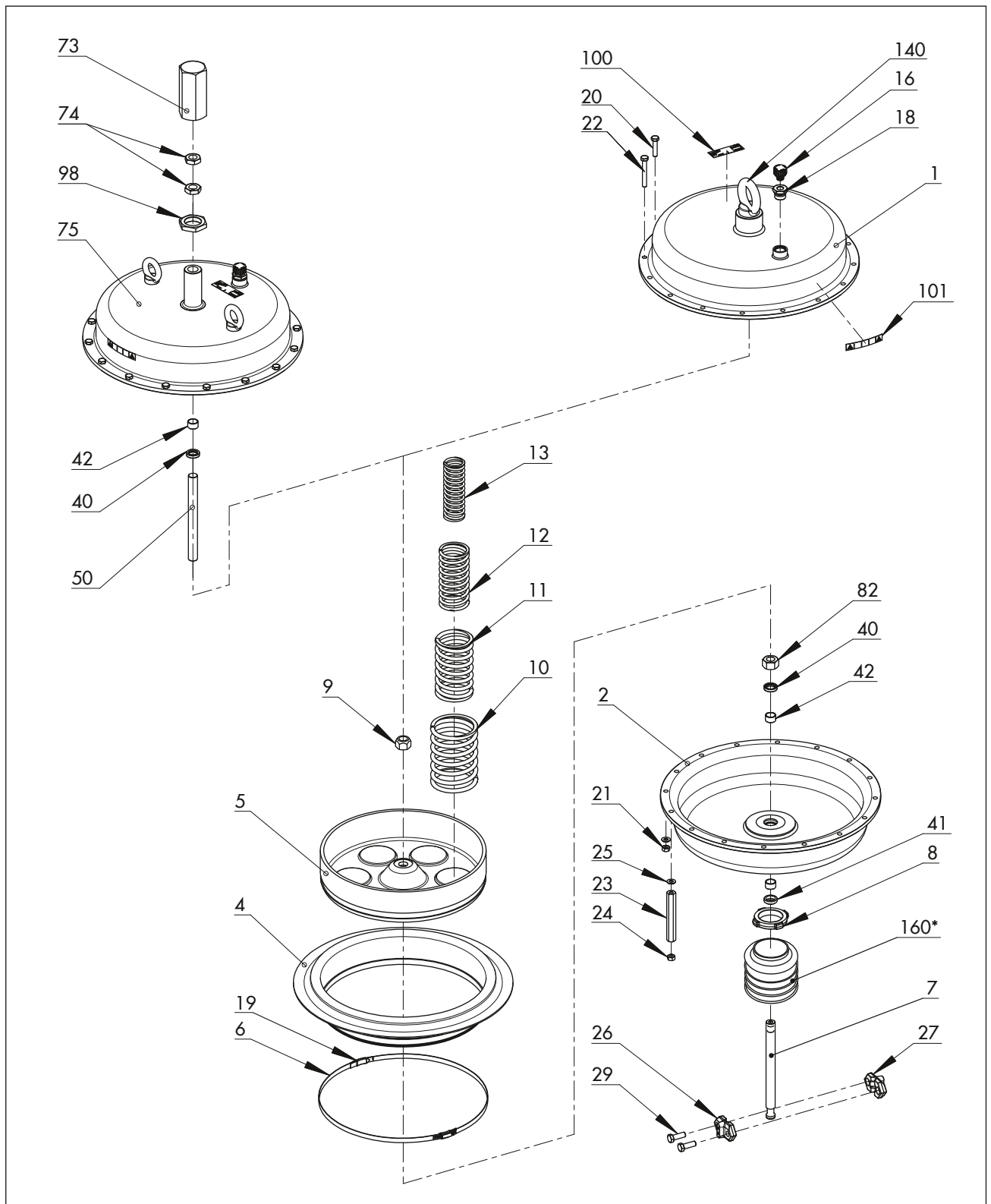
Fig. 19: Accionamiento Tipo 3271, 1400-60 cm 2
