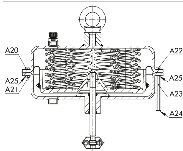
Fig. 10: Accionamiento con tornillos y tuercas tensores (ejemplo)
