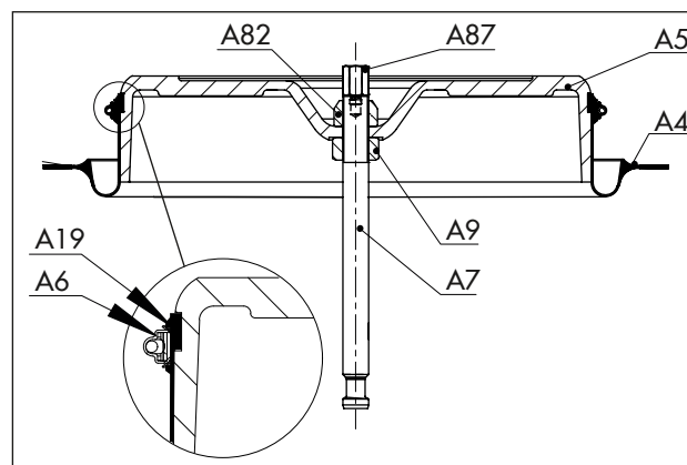
Fig. 15: Disposición de las piezas, sentido de actuación FE (1400-60 cm 2 )
