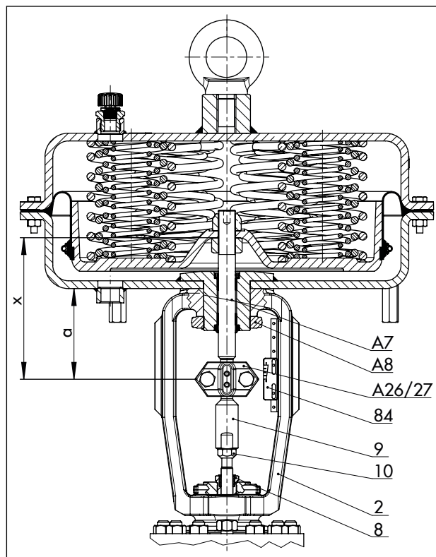
Fig. 8: Accionamiento neumático Tipo 3271 montado en una válvula lineal
