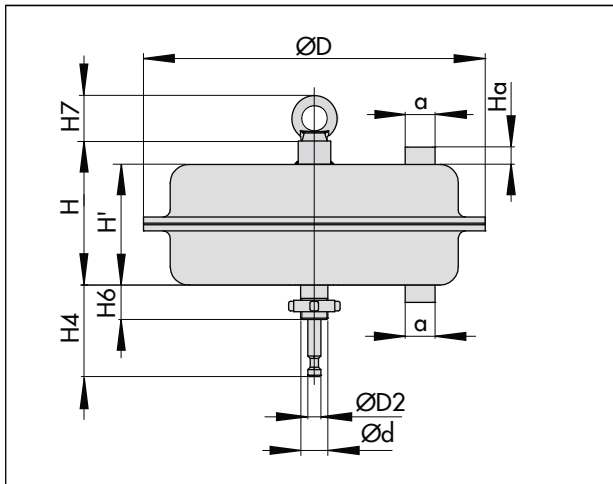
Fig. 3: Tipo 3271 con superficie de accionamiento 1400-60 cm 2
