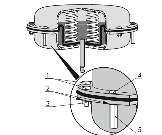
Fig. 18: Resortes pretensados (esquema)
