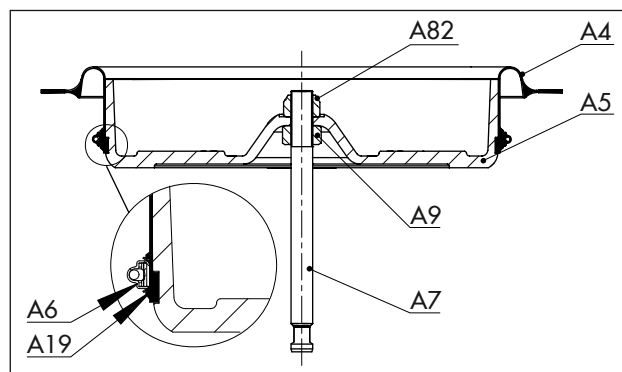
Fig. 13: Disposición de las piezas, sentido de actuación FA (1400-60 cm 2 )
