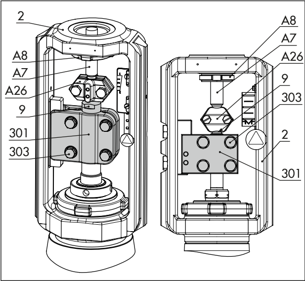
Fig. 9: Seguro anti rotación: ejecución estándar en el lado izquierdo, ejecución especial en el lado derecho
