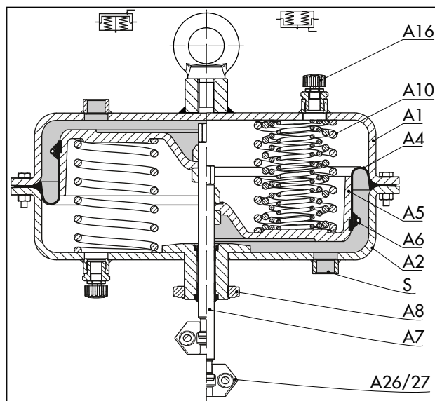
Fig. 12: Accionamiento neumático Tipo 3271, ejemplo con superficie de 1400-60 cm 2
