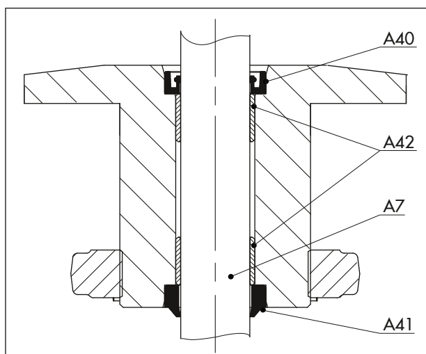
Fig. 17: Tipo 3271 Junta del vástago del accionamiento
