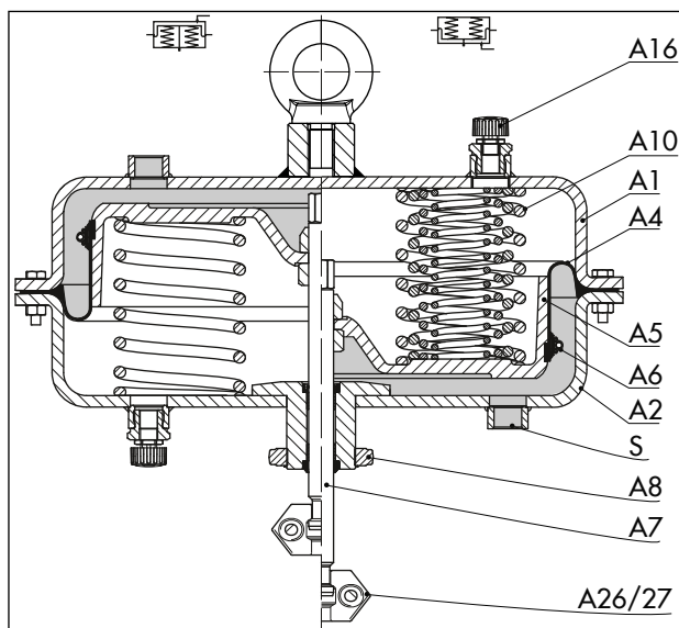
Fig. 2: Accionamiento neumático Tipo 3271, ejemplo con superficie de 1400\text{-}60 \text{ cm}^2
