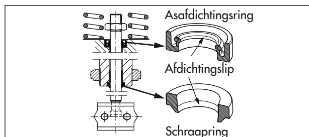
Afbeelding 14: Uitlijning asafdichtingsring en schraapring
