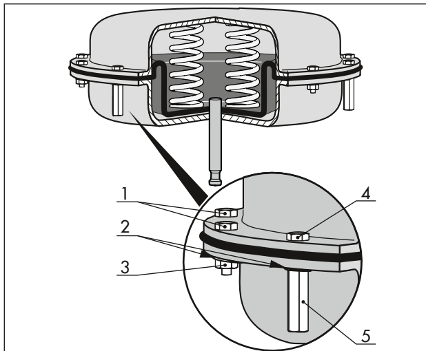
Afbeelding 16: Voorgespannen veren (schematische weergave)
