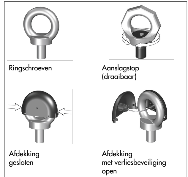
Afbeelding 5: Verliesbeveiliging aan ringschroeven/aanslagstop
