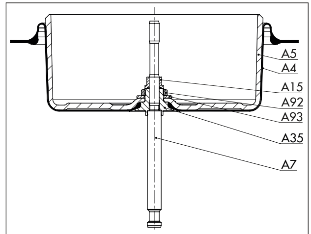
Afbeelding 12: Plaatsing van de componenten voor de werkingsrichting FA (1000 cm 2 )
