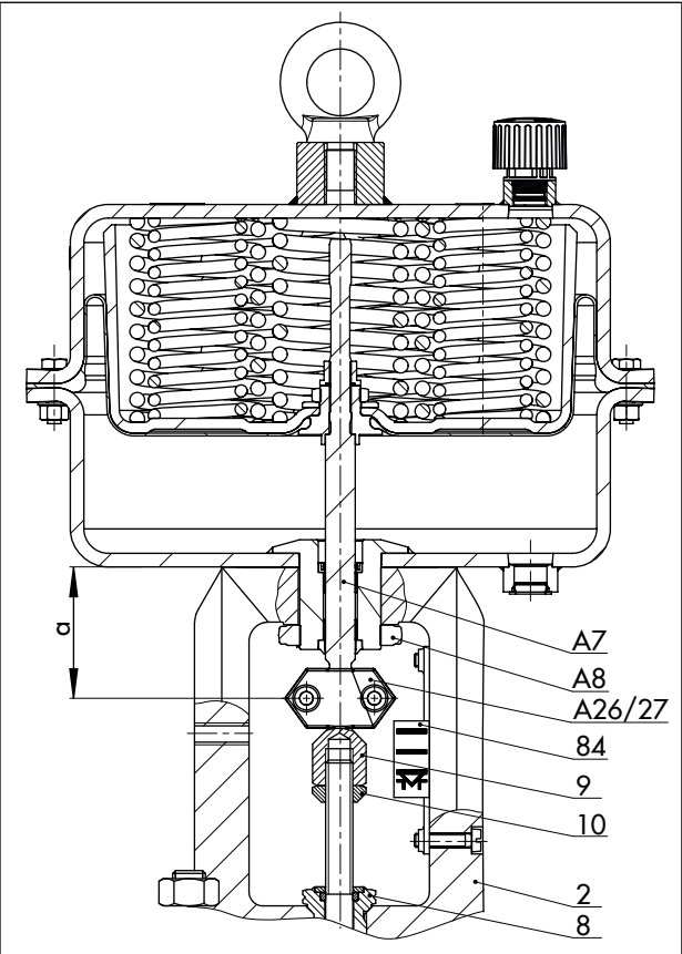
Afbeelding 8: Pneumatische aandrijving typ 3271 wordt op de slagventiel aangebouwd
