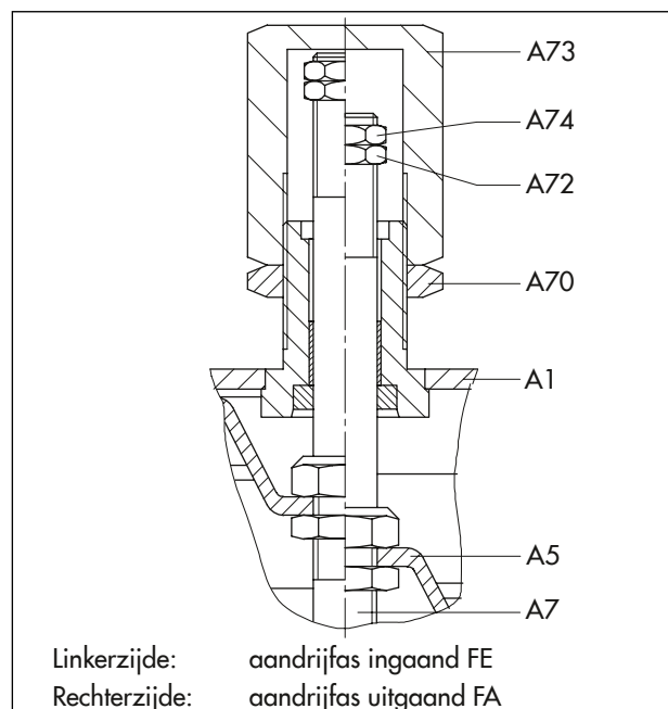
Afbeelding 11: Slagbegrenzing
