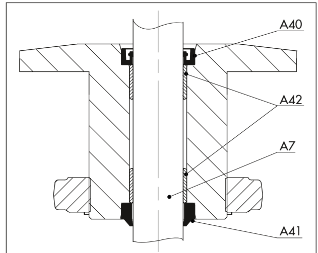
Afbeelding 15: Type 3271 afdichting aandrijf-as
