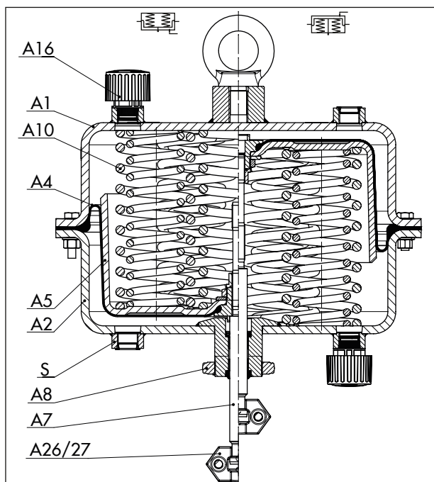
Afbeelding 2: Pneumatische aandrijving van het type 3271, voorbeeldafbeelding met een aandrijvingsoppervlak van 1000 \text{ cm}^2
