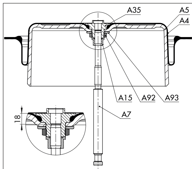
Afbeelding 13: Plaatsing van de componenten voor de werkingsrichting FE (1000 cm 2 )
