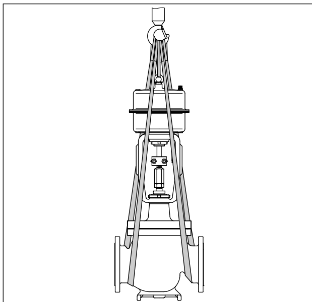
Afbeelding 7: Hefpunten op het regelventiel (voorbeeld)
