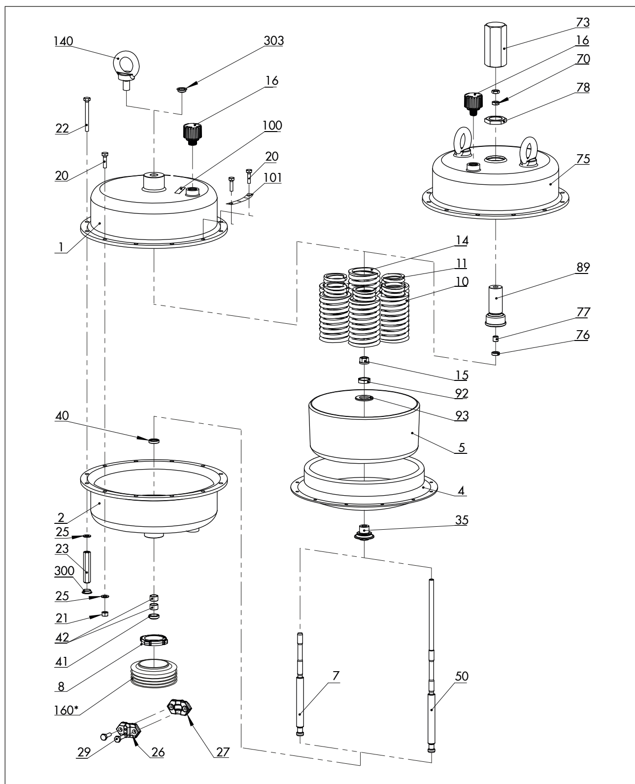
Afbeelding 17: Aandrijving van het type 3271, 1000 cm 2
