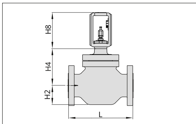
Fig. 6: Tipo 3251/3251-AM hasta DN 80/NPS 3 sin base
