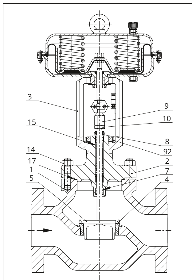
Fig. 23: Tipo 3251/3251-AM en ejecución estándar con accionamiento Tipo 3271
