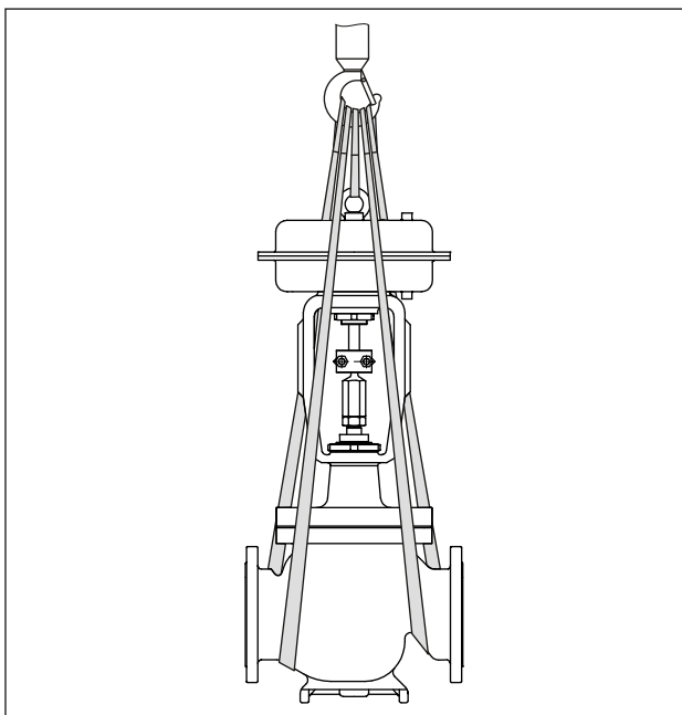
Fig. 11: Puntos de elevación en la válvula con eslinga adicional en el accionamiento
