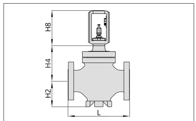
Fig. 7: Tipo 3251 a partir de DN 100/NPS 4 con base
